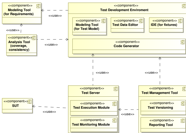
Abbildung 2: Telling TestStories Framework
