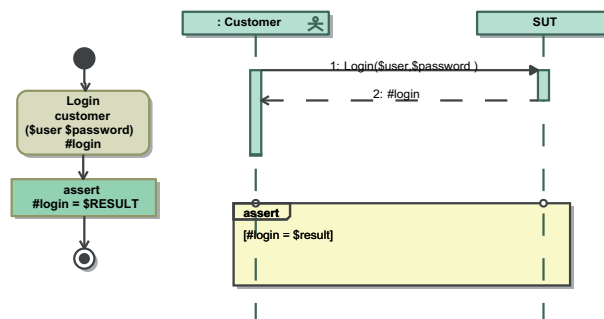
Abbildung 1: Test Story für einen Login–Vorgang als Aktivitäts- und Sequenzdiagramm
